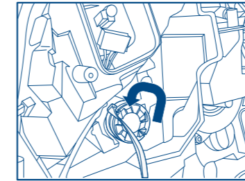
3 Ortadaki halkayı çıkarın ve tutucuya takın. Metal klipsle halkayı sabitleyin. Ampülü tutucuya takın. Sabitlemek için ampülü dikkatlice çevirin.
