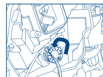
3 Извлеките центральное кольцо и установите его в держатель. Закрепите его металлическим зажимом. Установите лампу в держатель. Аккуратно поверните лампу для фиксации.
