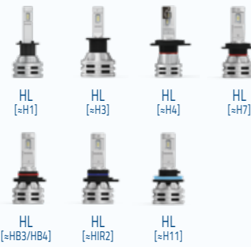
БЛИЖНИЙ СВЕТ ДАЛЬНИЙ СВЕТ
