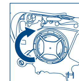
6 Закройте крышку фары.
