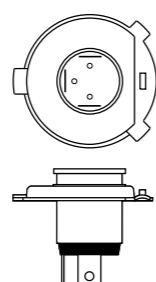
P43t 7004-39
