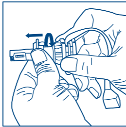
3 أخرج الحلقة الوسطى وربّب المصباح في الحامل. ثبّت الحلقة بإحكام بواسطة المشبك المعدني. ركب اللمبة في الحامل. قم بتدوير اللمبة بلطف لتثبيتها بإحكام.
