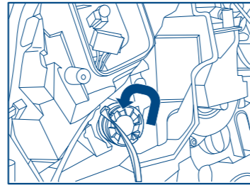
3 أخرج الحلقة الوسطى وربّب المصباح في الحامل. ثبّت الحلقة بإحكام بواسطة المشبك المعدني. ركب اللمبة في الحامل. قم بتدوير اللمبة بلطف لتثبيتها بإحكام.
